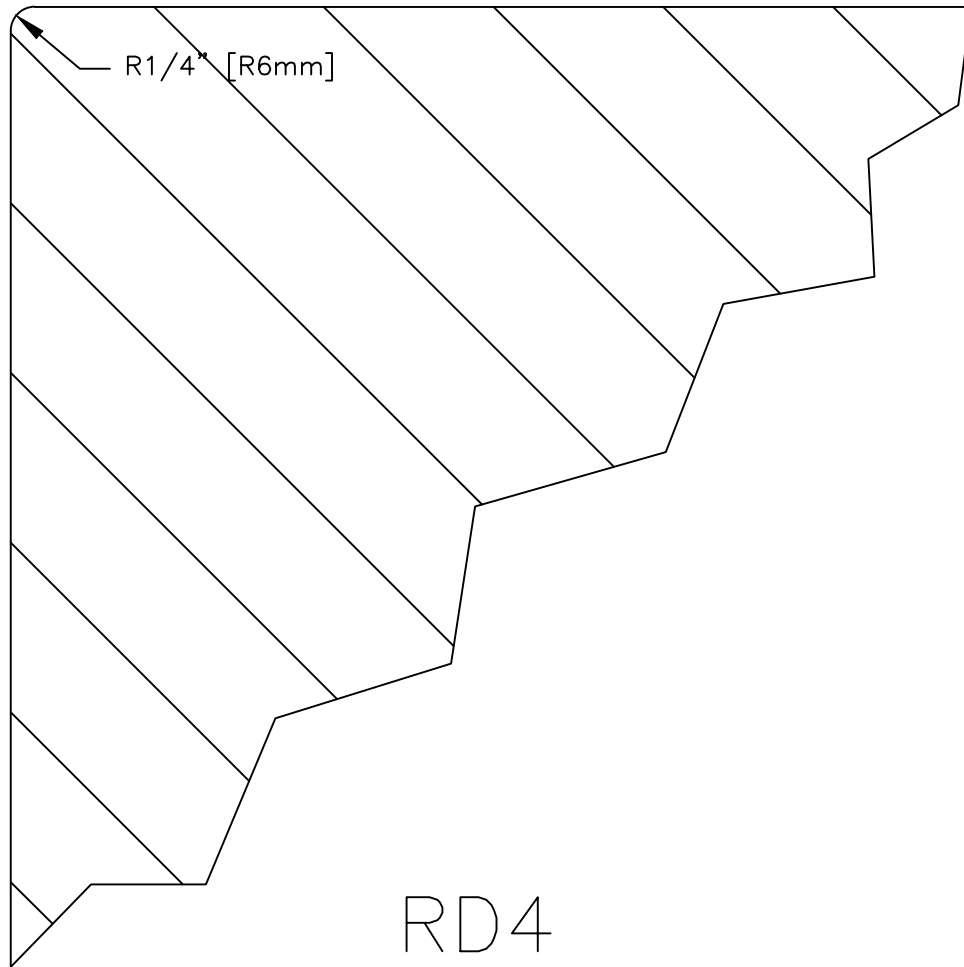
RD4 1/4" RADIUS EDGE SECTION
