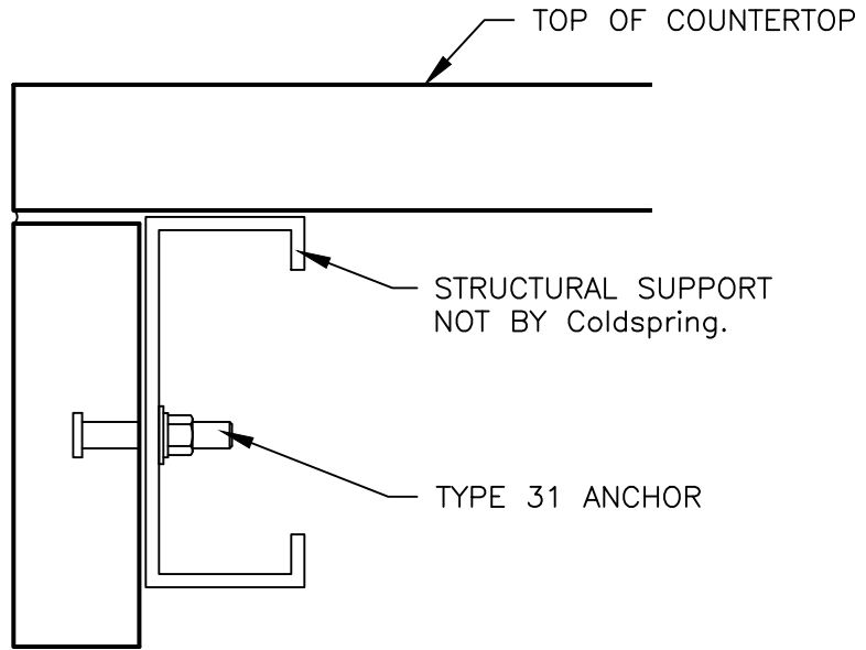
APRON SECTION
