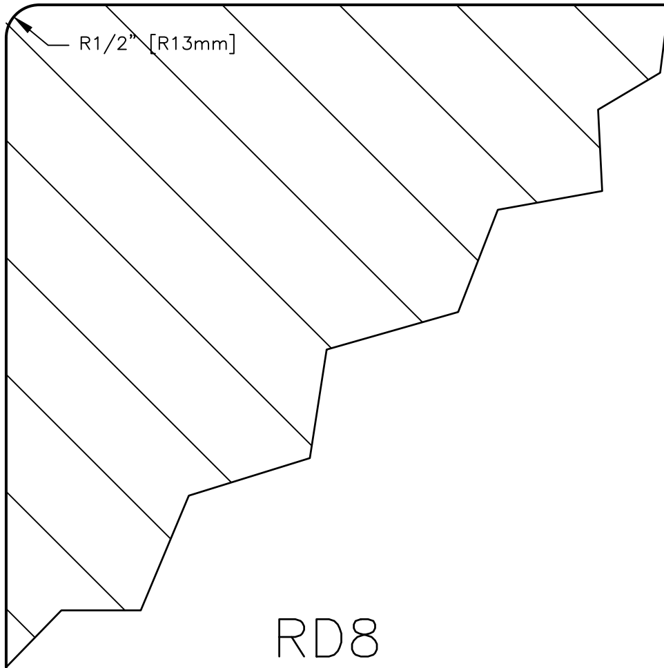
1/2" RADIUS EDGE SECTION
