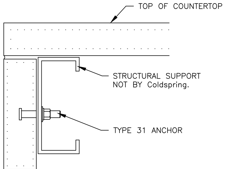
APRON SECTION
