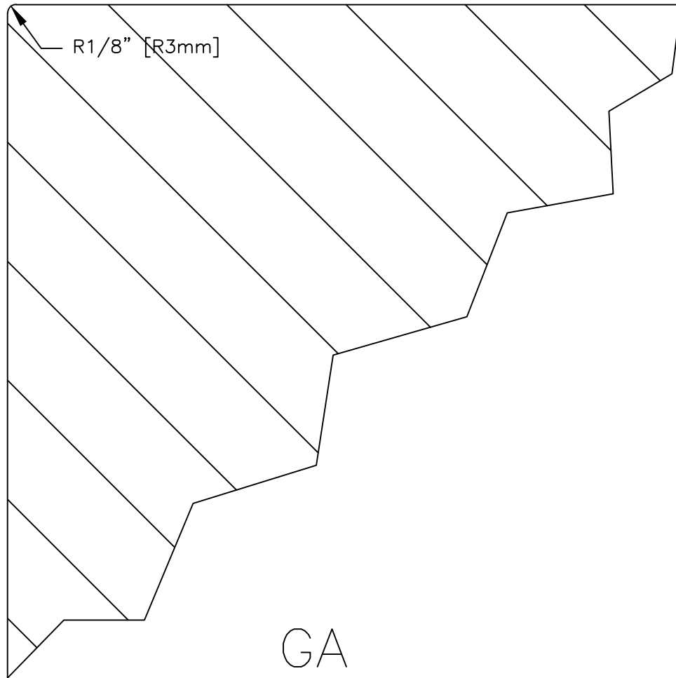
1/8" RADIUS EDGE SECTION
