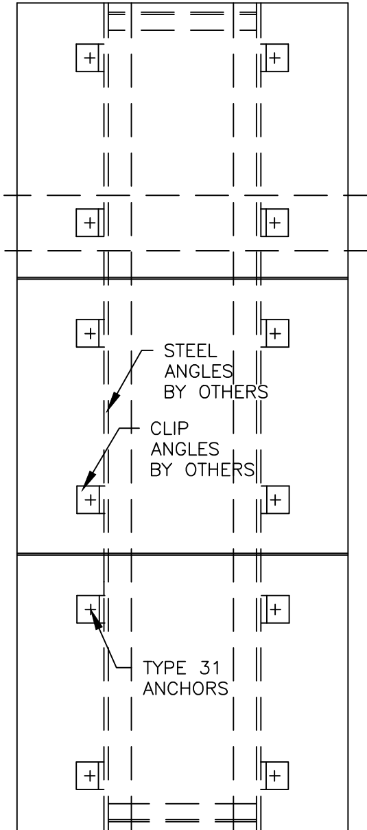
ELEVATION
